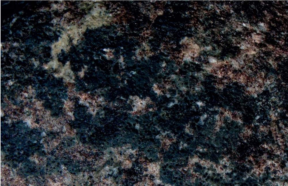
Abb. 1: Lager von Verrucaria madida (gesammelt während der Dürreperiode im Jahr 2003). Fig. 1: Thallus of Verrucaria madida (collected during the drought period in 2003).
